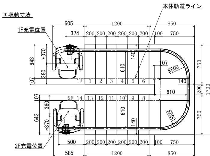
(階段平面図)
