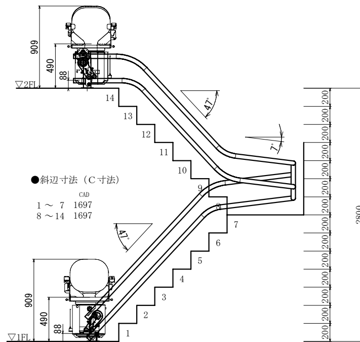
(階段立面図)
